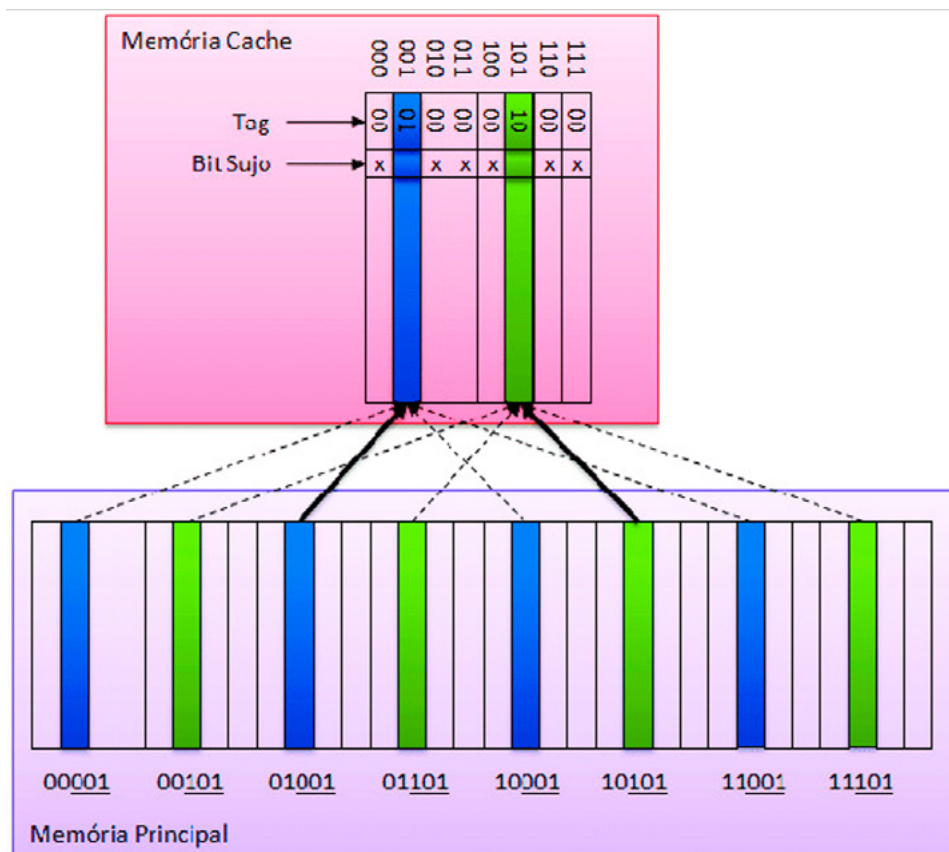
Figura 3: Mapeamento Direto
